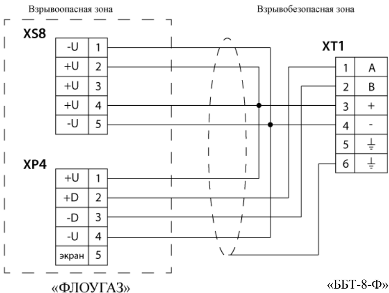
Рисунок 2. Схема подключения блока к корректору «ФЛОУГАЗ».
